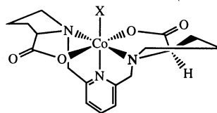
\Delta -[Co(( R,R )-promp)X] +
