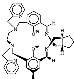
S,S -cypim
